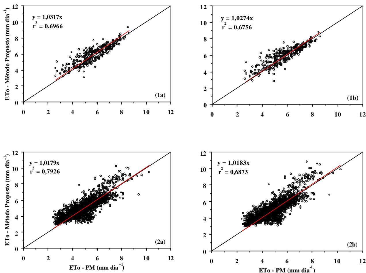
Figura 1. Relação entre a ETo diária estimada pelo método de Penman - Monteith (Eto-PM) e pelos métodos propostos, com (a) e sem (b) o termo \Delta s^2 , para Parnaíba (1) e Teresina (2), PI.
